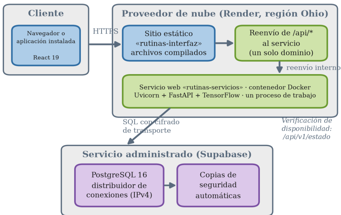
Figura 31. Diagrama de arquitectura técnica y despliegue del sistema
