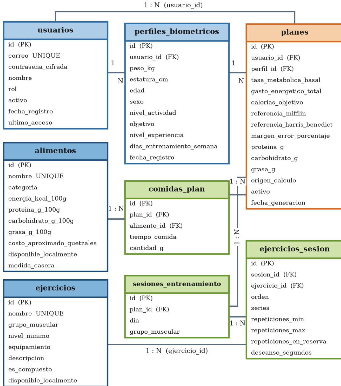
Figura 35. Modelo entidad-relación del sistema, primera parte
