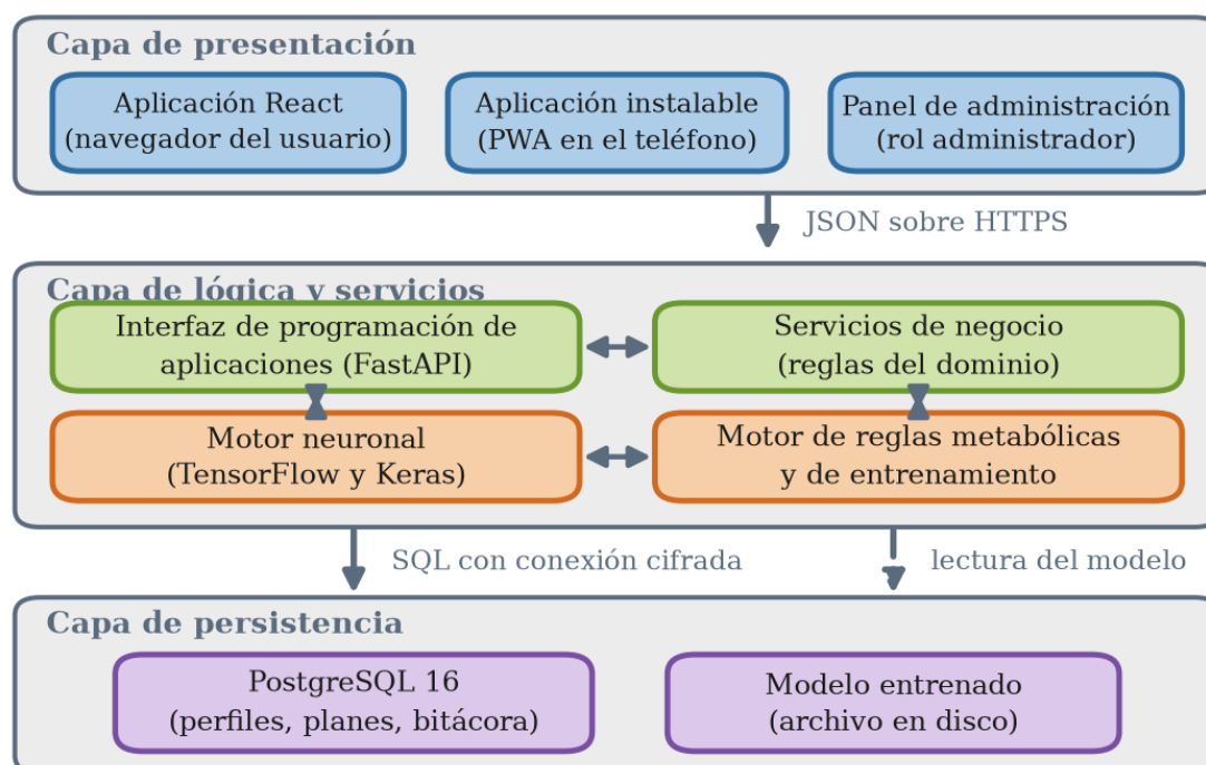
Figura 29. Vista general de la arquitectura en tres capas del sistema
